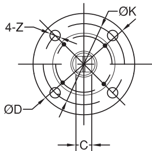
TOP FLANGE
