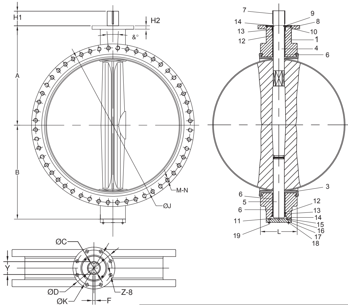
TOP FLANGE
