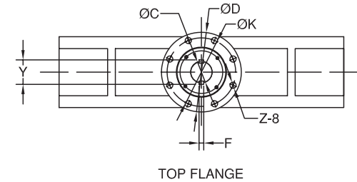
TOP FLANGE
